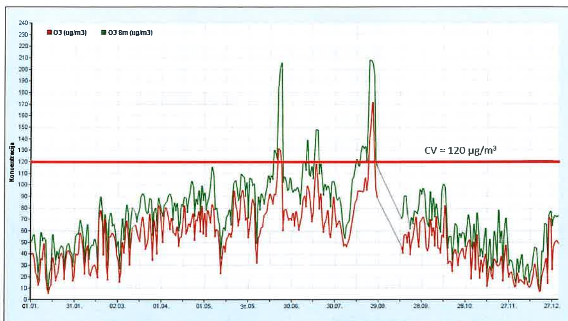
Slika 5. Grafički prikaz srednjih dnevnih vrijednosti i najviših dnevnih osmosatnih srednjih vrijednosti prizemnog ozona \text{O}_3 na mjernoj postaji Mirogojska cesta
