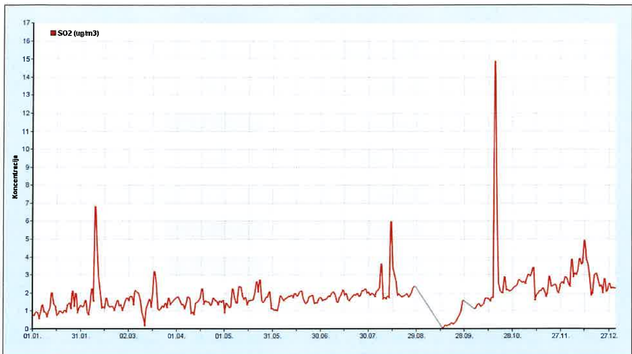
Slika 3. Grafički prikaz 24-satnih koncentracija sumporovog dioksida SO 2 na mjernoj postaji Mirogojska cesta
